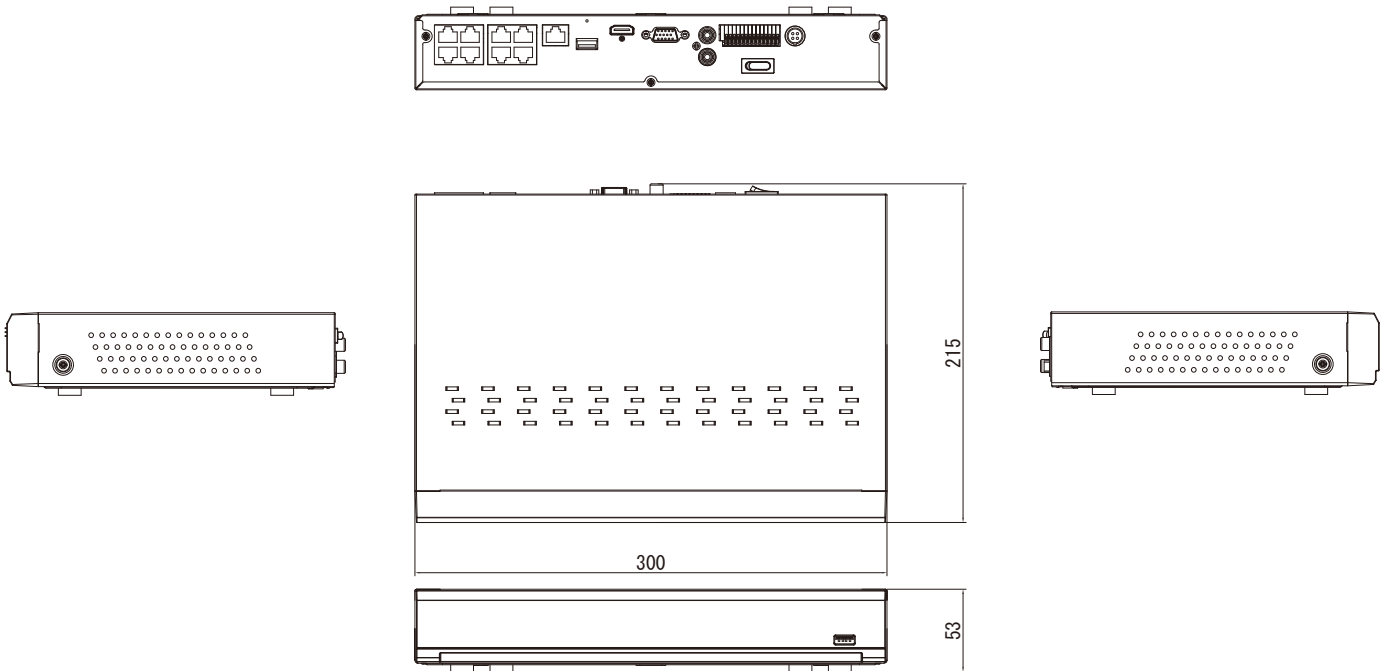
寸法図
