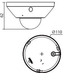
■外形寸法(mm)
