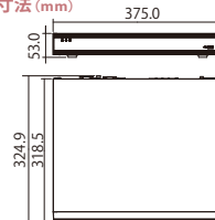
■ 外形寸法 (mm)
