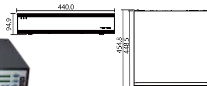
■ 外形寸法 (mm)
