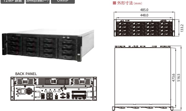
■ 外形寸法 (mm)
