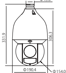
■外形寸法(mm)
