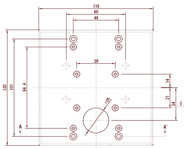
寸法図(mm)
