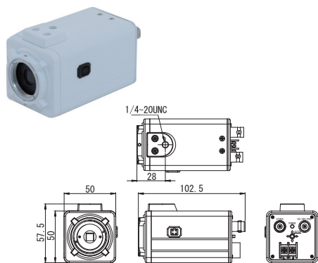
■ 寸法図 (mm)
