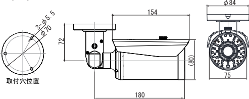
■ 寸法図 (mm)
