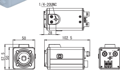
■ 寸法図 (mm)
