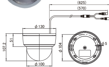
■ 寸法図 (mm)
