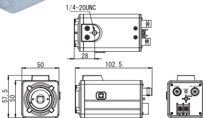
■ 寸法図 (mm)
