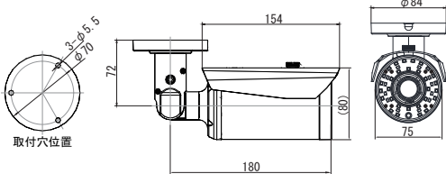
■ 寸法図 (mm)
