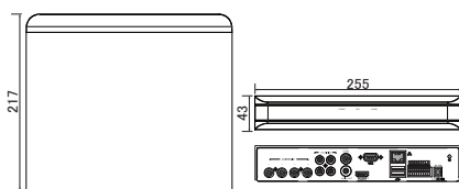
■寸法図 (mm)
