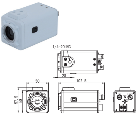
■ 寸法図 (mm)
