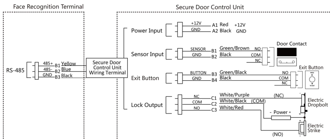
図4-2 安全ドアコントロールユニットの配線
