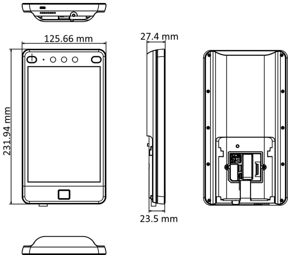
図D-1 寸法
