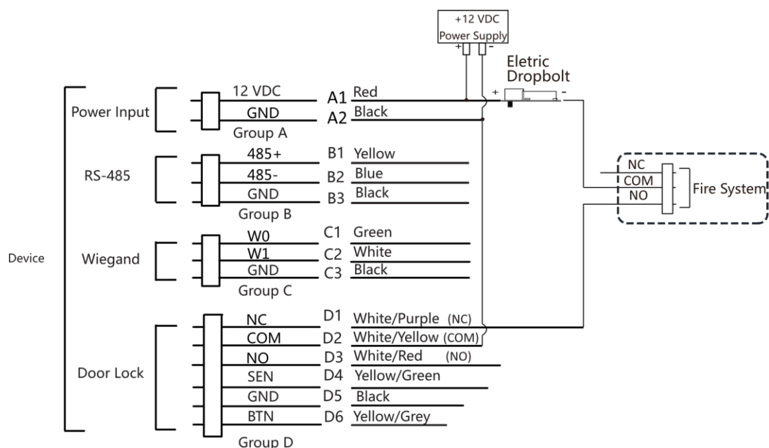
図4-5 配線デバイス
