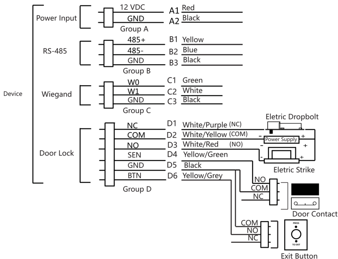
図4-1 機器の配線図
