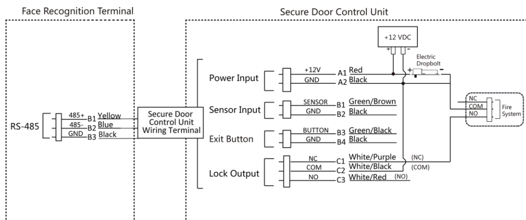
図4-6 セキュア・ドア制御ユニットの配線
