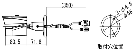
取付穴位置
