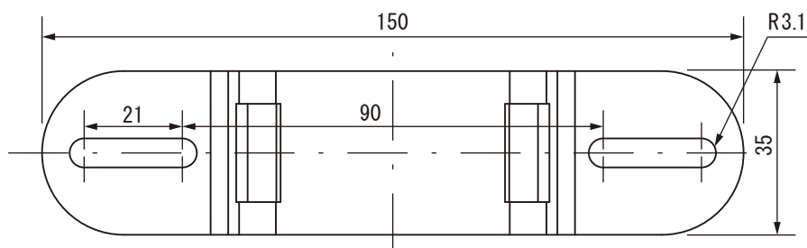
(上面図)
