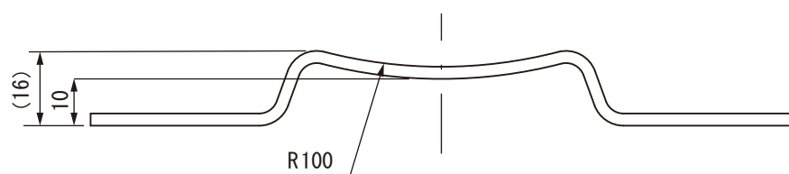
(側面図)
