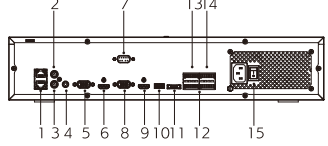
■背面端子図
