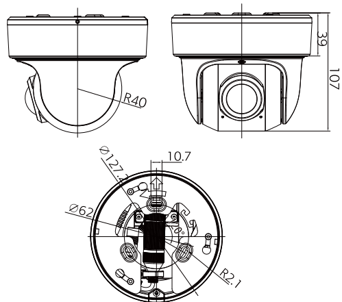
■寸法 (単位mm)
