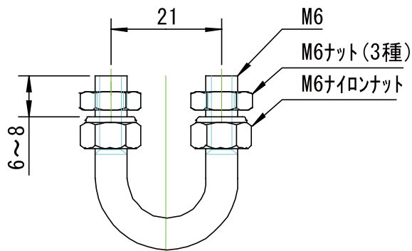
鋼管用ステンレスUボルト M6-8A
