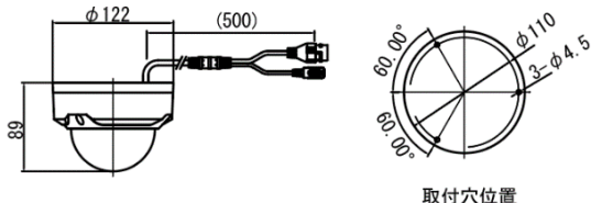
取付穴位置
